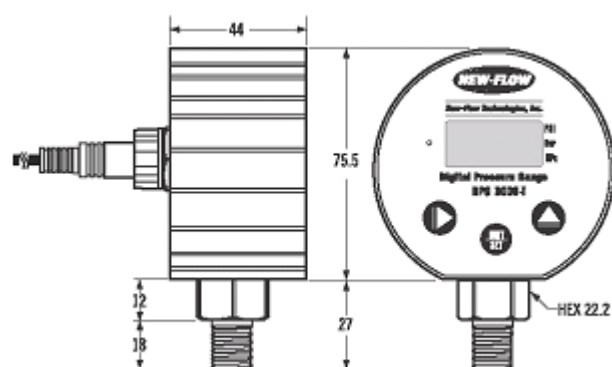
Dimensioni
