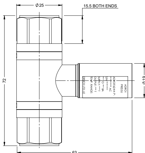
Costruzione per campi differenziali
