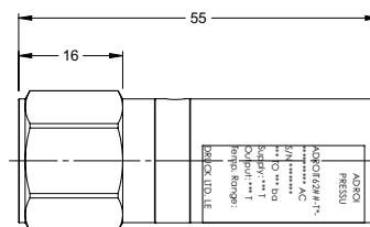
Costruzione per campi medi (campi di pressione > 10 BAR A > 350 BAR)
