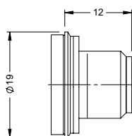
Connettore M12x1 4-PIN per alta temperatura (TD)
