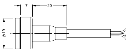
CAVO IN POLIURETANO / RAYCHEM
