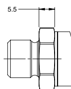
Attacchi di pressione maschi
