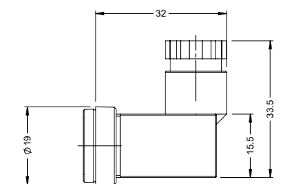
Connettore MICRODIN (PASSO 9,4 MM)
