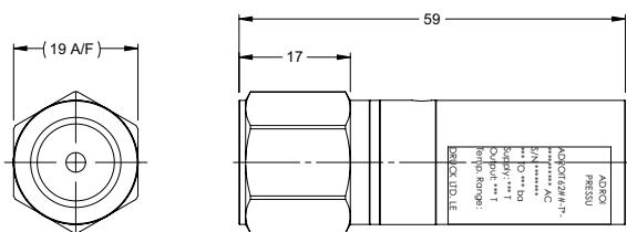
Costruzione per basse pressioni (campi di misura <10 BAR)
