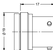
Connettore a BAIONETTA MIL-C-26482 PER TEMPERATURA STANDARD (TB)
