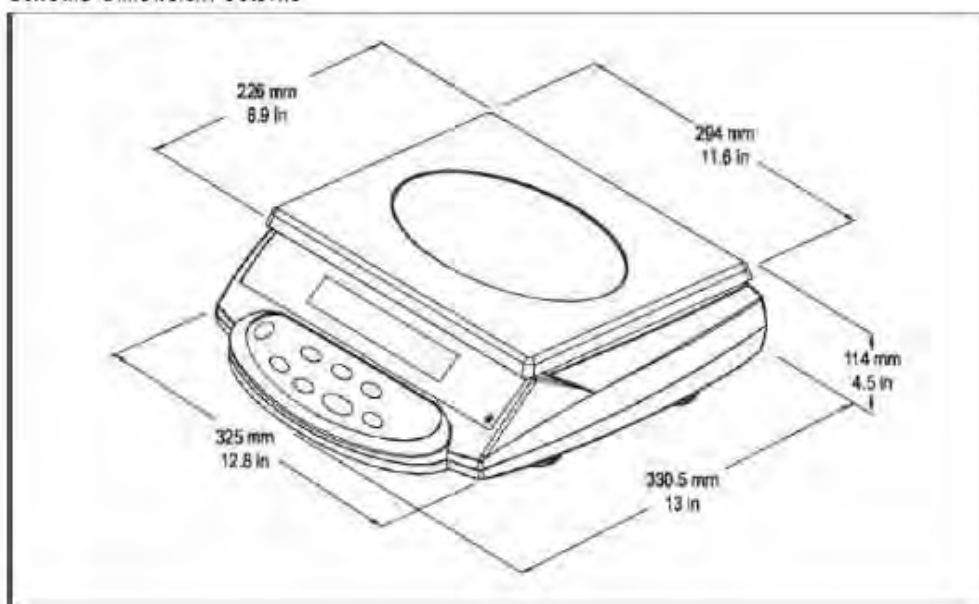
Schema dimensioni esterne
